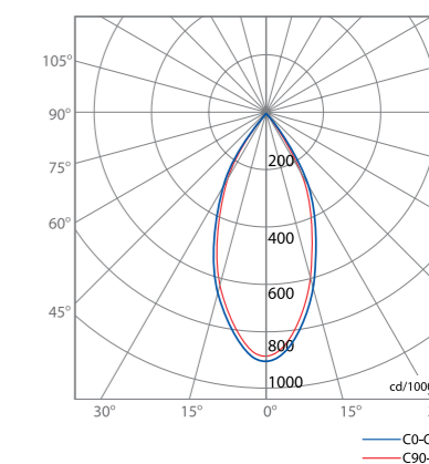
Диаграмма направленности АНЛ 30°
