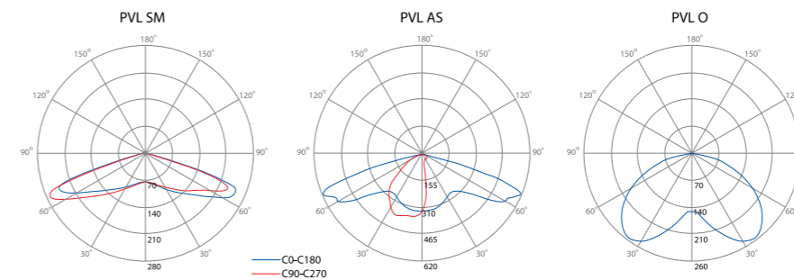
Диаграммы направленности
